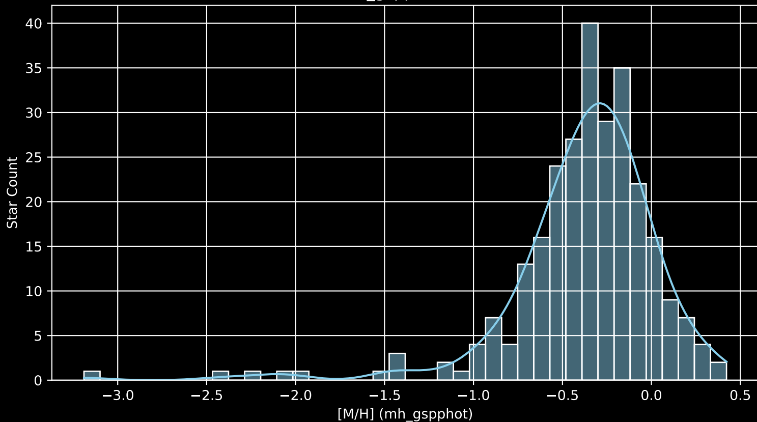
GALAH DR4 Field: [9158] [M/H] (mh_gspphot) (n= 271)
