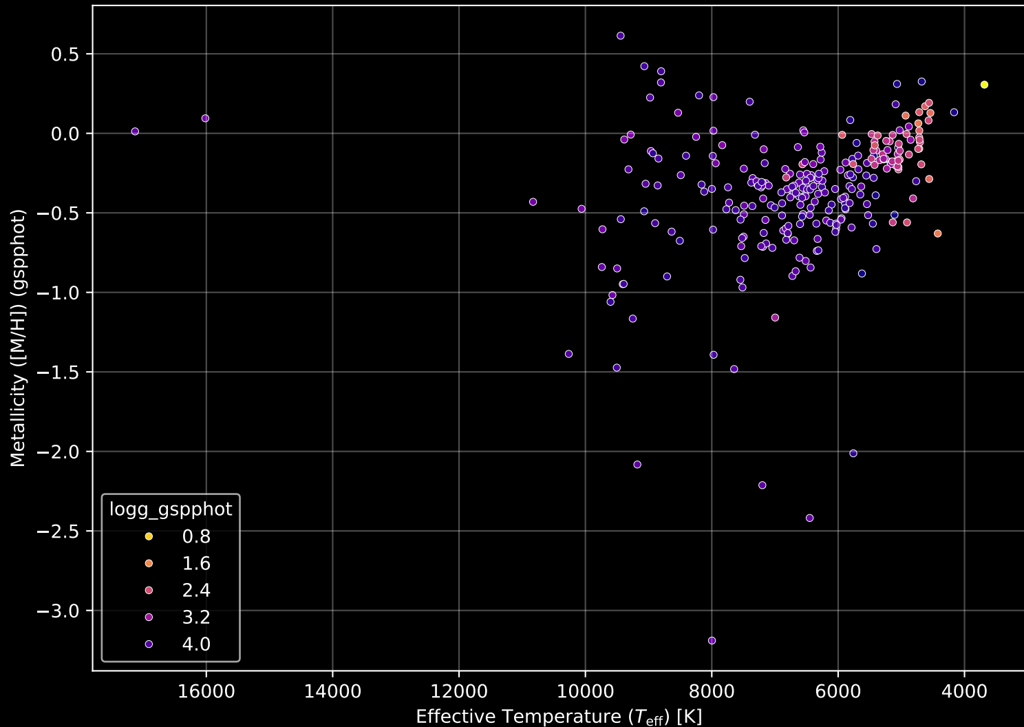
GALAH DR4 Field: [9158] Stellar Population Parameters (n= 272)
