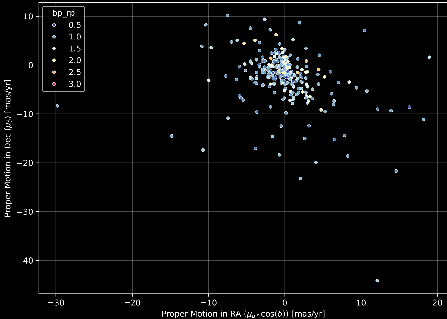
GALAH DR4 Field: [9158] Proper Motion Diagram (n= 272)
