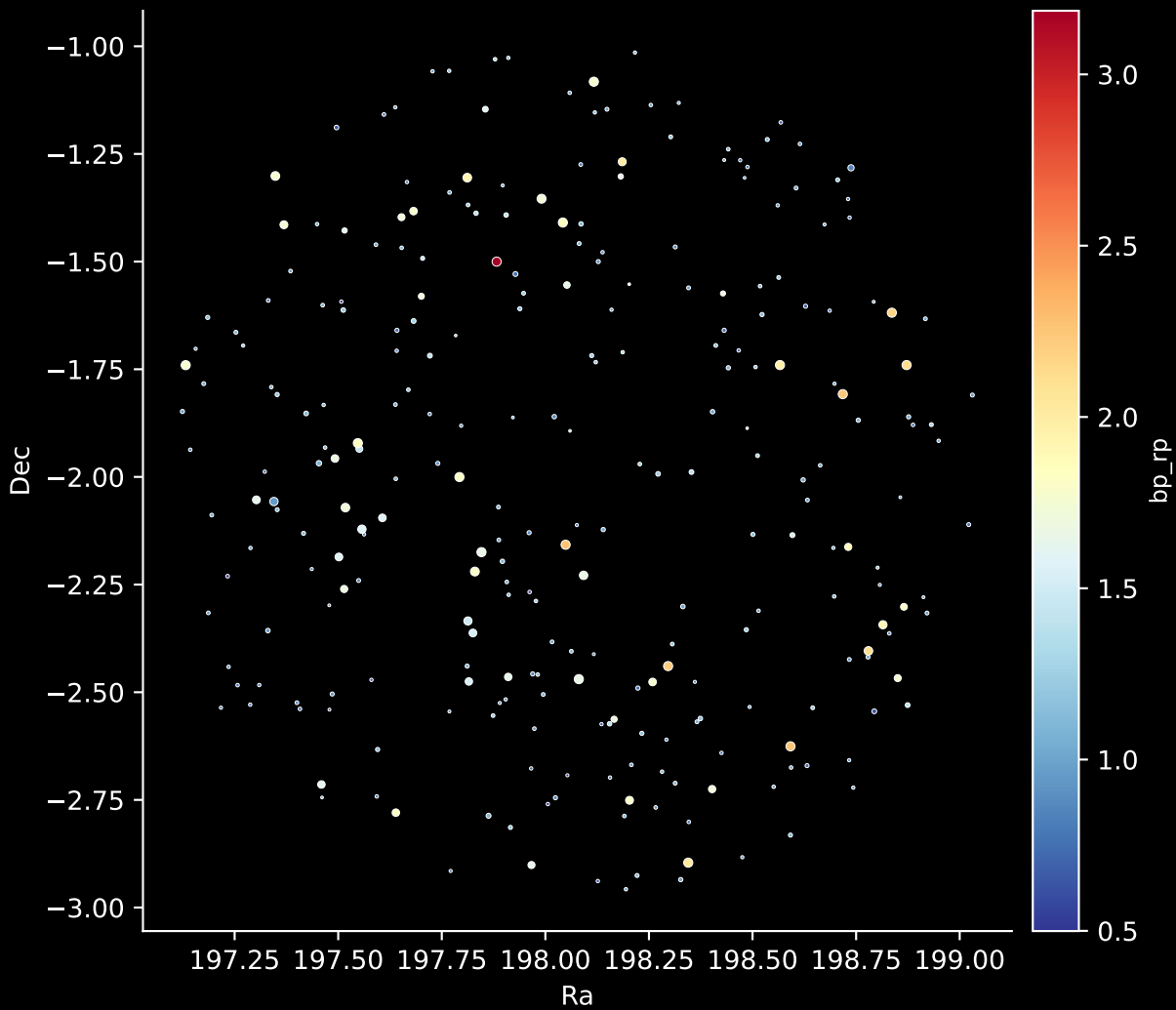
GALAH DR4 Field: [9158] Stars: 272
