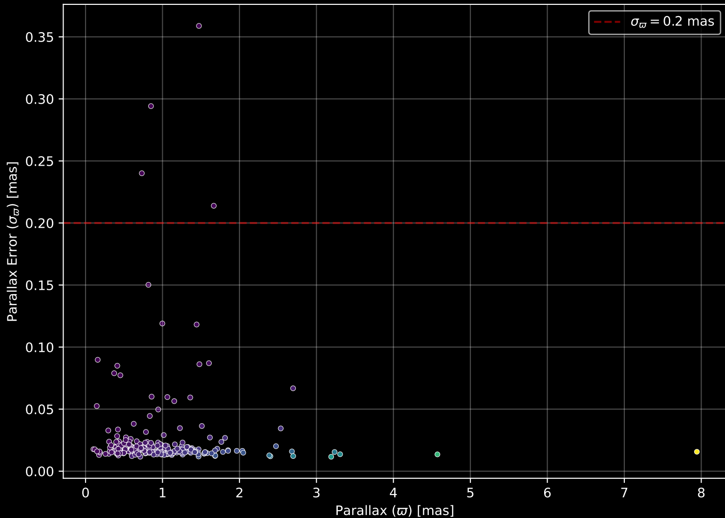
GALAH DR4 Field: [9158] Parallax Quality (n= 272)
